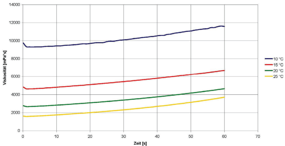
Diagramm 1: Mischungsviskosität der Harzsysteme "Trelleborg Epoxy HC120 (A+B)" und "Trelleborg Epoxy HC120+ (A+B)"
