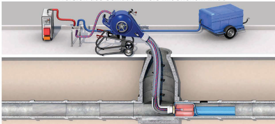
Schlauchlinier vom Inversionsstutzen trennen, Kalibrierschlauch einführen und am Startpunkt positionieren
