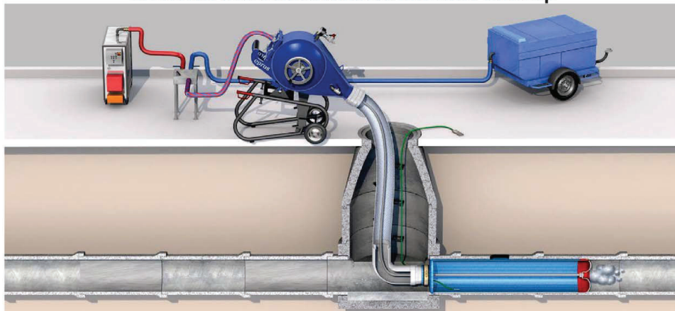
Aushärtung mit Liner EndCap: Heißes Medium wird zum Schlauchlinterkopf geführt und strömt im Schlauchlinter zurück. Alternativ: Mit Dampfauslassventil strömt das Dampf-/Luftgemisch in Inversionsrichtung durch den Schlauchlinter und tritt am Schlauchlinterkopf aus
