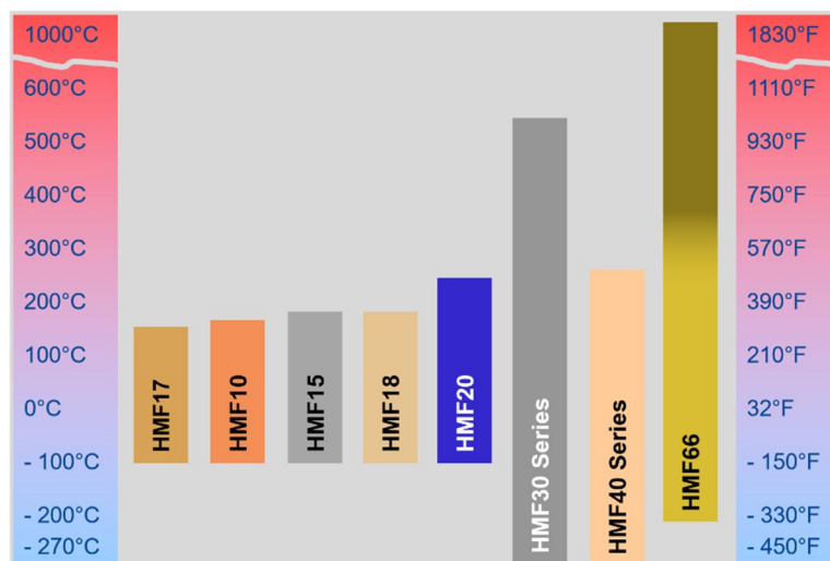
Orientierung der Anwendungstemperaturbereiche
